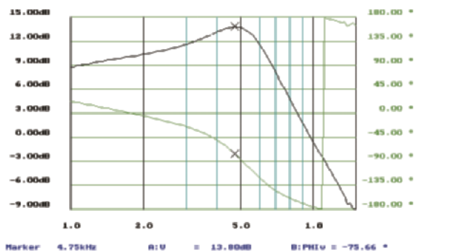
Messdiagramm: Gibson 1953 P-90
